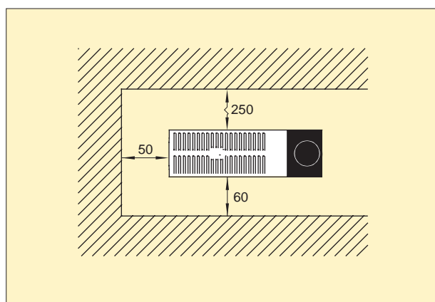
Рисунок 1: Минимальные расстояния при установке.
